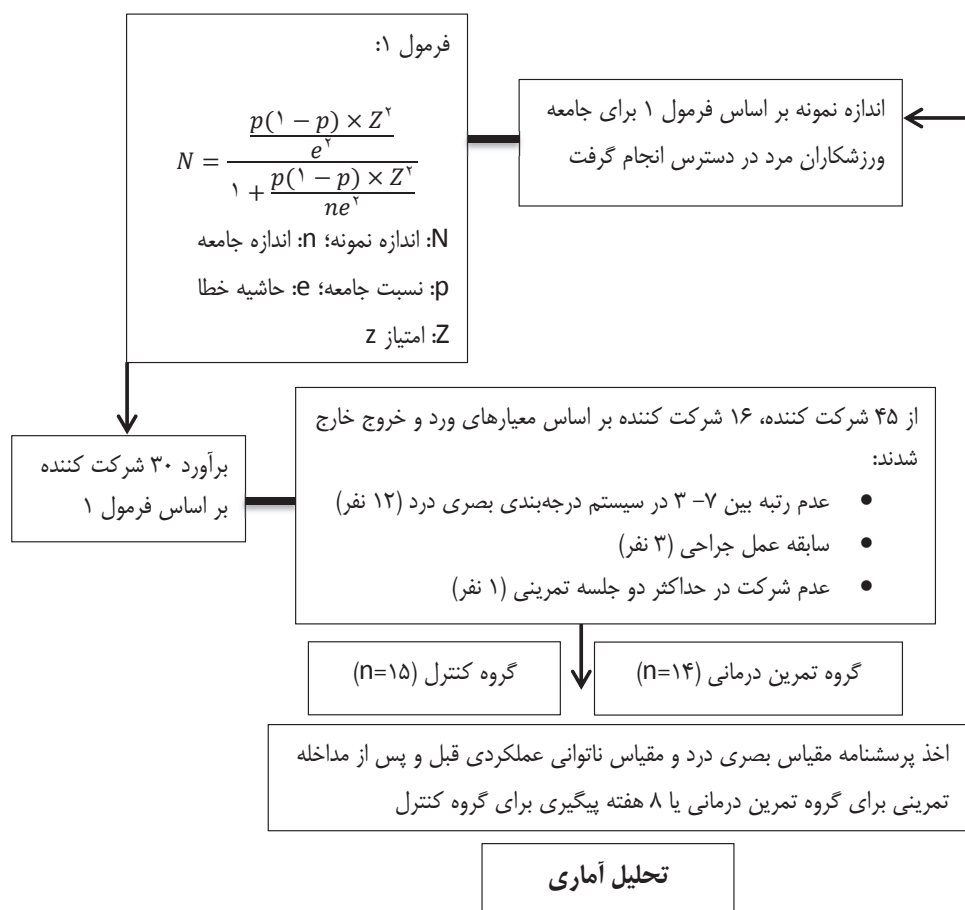
شکل ۱. فلوجارت مطالعه
