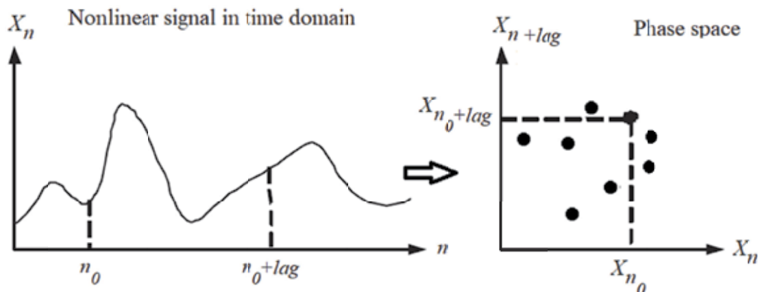
شکل ۲: نمایشی از بازسازی فضای فاز. طرح پوانکاره یک رویکرد تحلیلی غیرخطی در صفحه دو بُعدی است که در آن یک سیگنال زمان‌بندی شده پس از یک تأخیر زمانی در برابر خودش رسم می‌شود.
